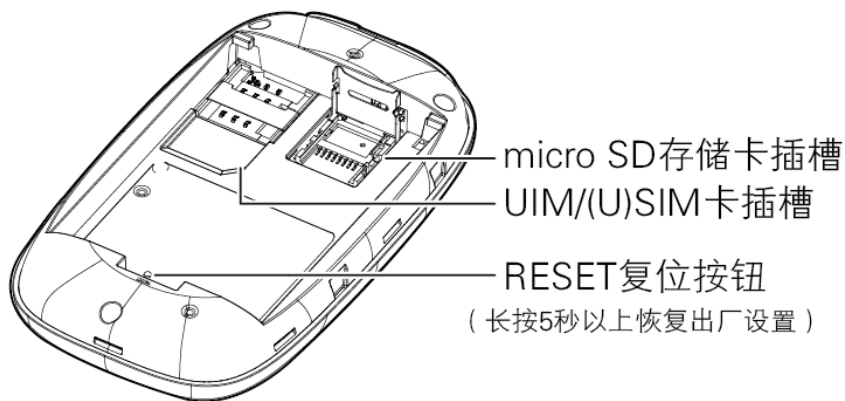
图 3.4 内部结构图
